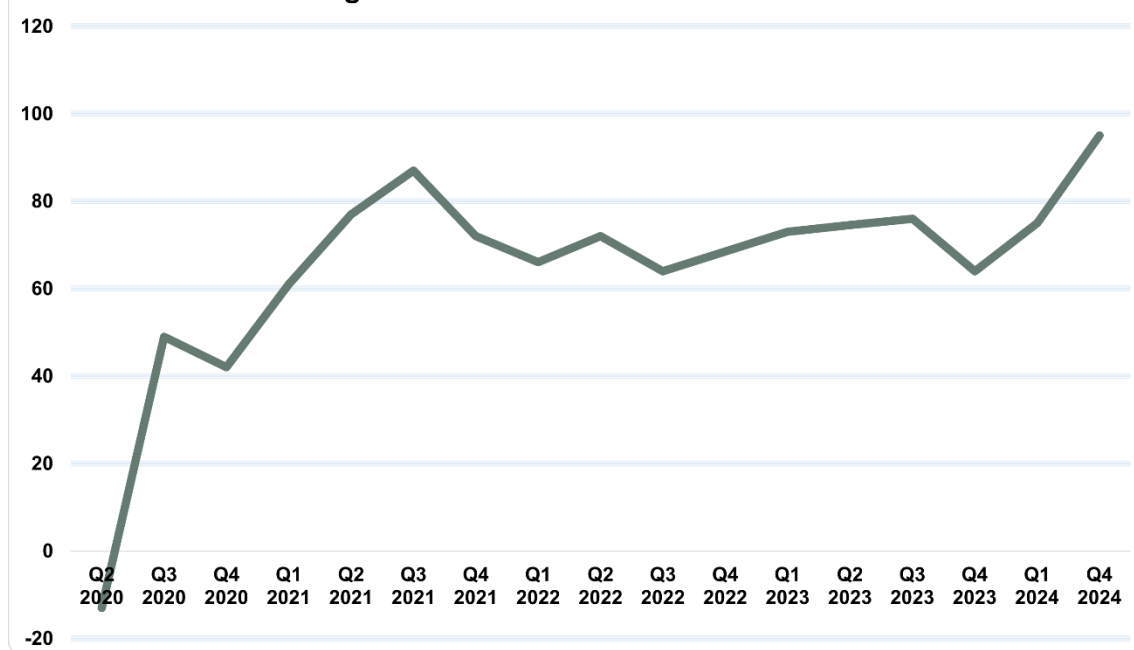
Figur 1. Konfidensindikator 2020-2024
